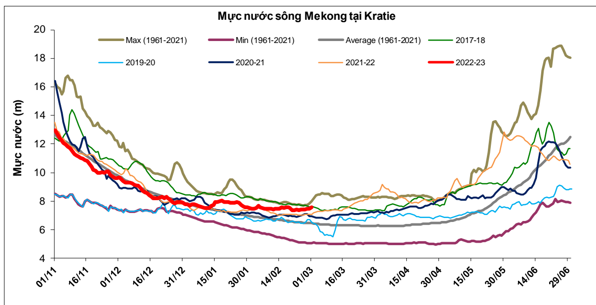
Hình 3. Diễn biến mực nước về qua trạm Kratie, cập nhật ngày 01/3/2023
