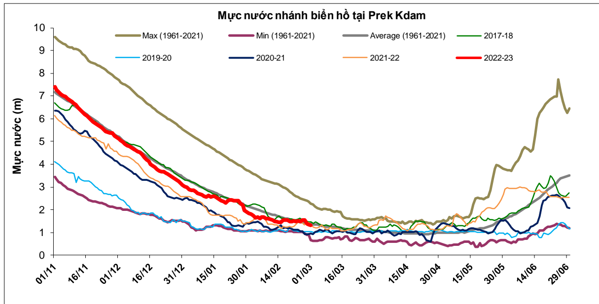
Hình 1. Diễn biến mực nước trạm Prek Kdam - Biển hồ, cập nhật ngày 01/3/2023
