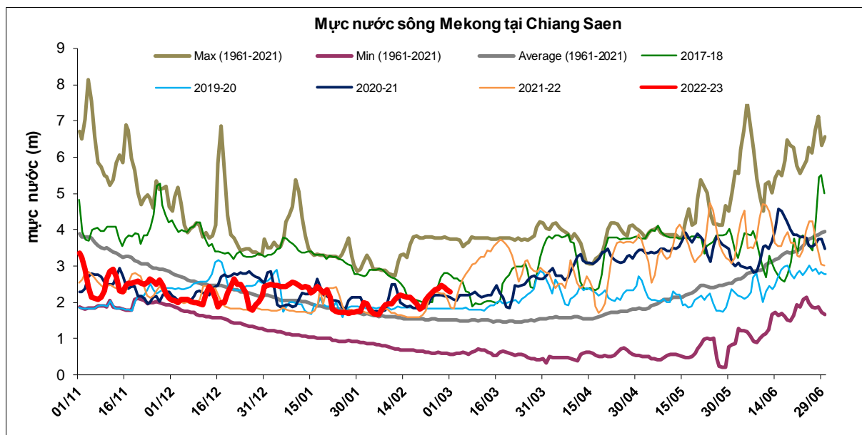
Hình 2. Diễn biến mực nước tại Chiang Saen –Thái Lan, cập nhật 01/3/2023
